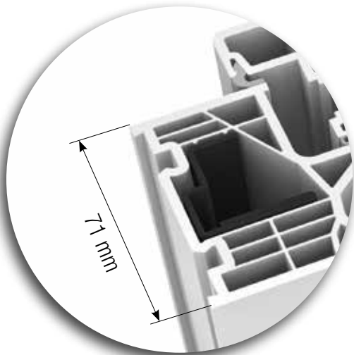
Bautiefe
