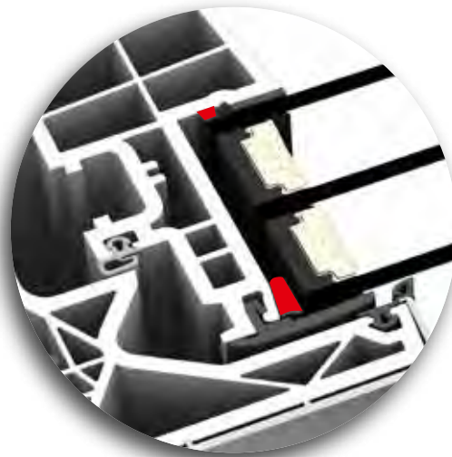
I-tec Verglasung
